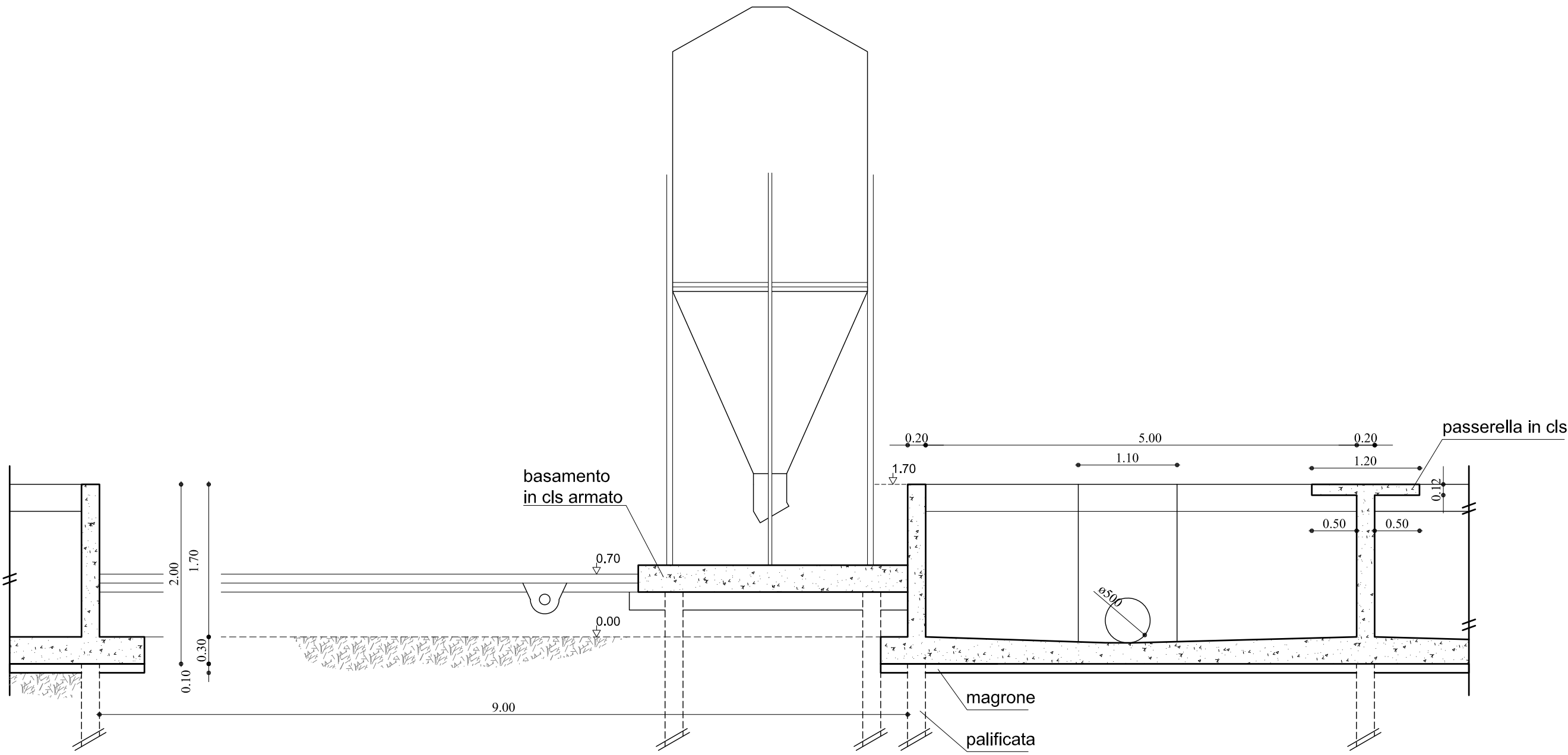
SEZIONE B-B
